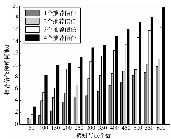
图 8 不同信任推荐个数的耗能比较
