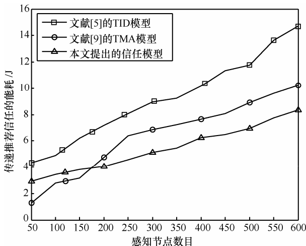
图 7 3 个不同信任模型的耗能比较
